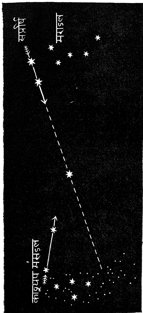
चित्र २—सप्तर्षि और कश्यप मराडल
